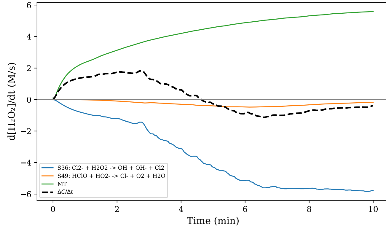
(d) \text{H}_2\text{O}_2
